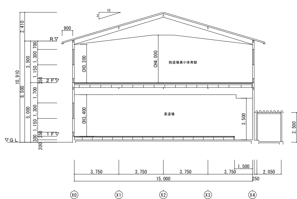
断面図 1/200
