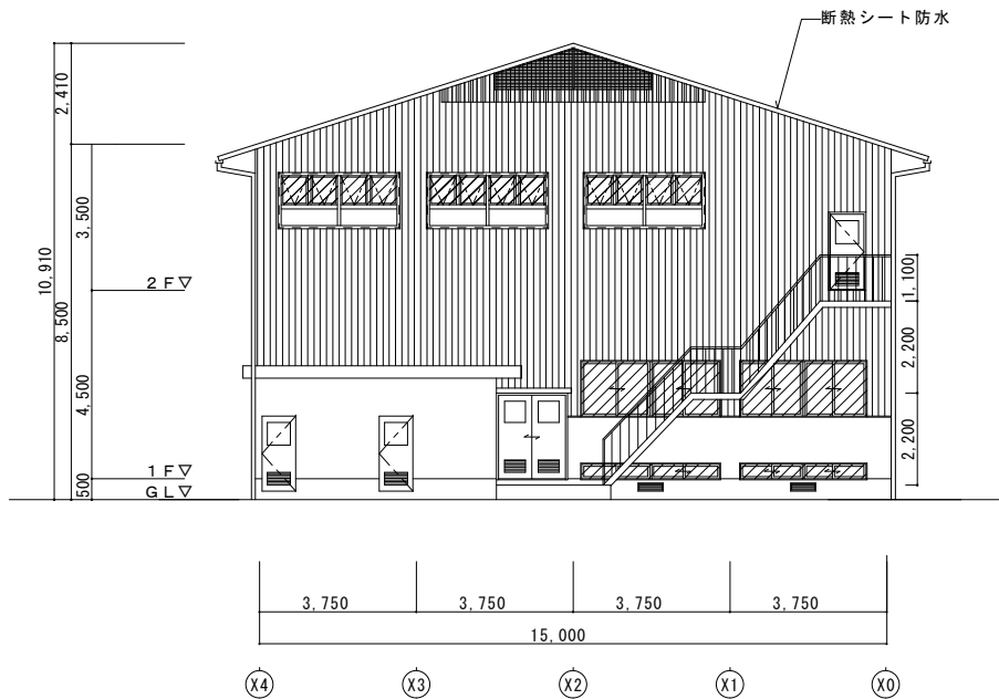
北側立面図 1/200
