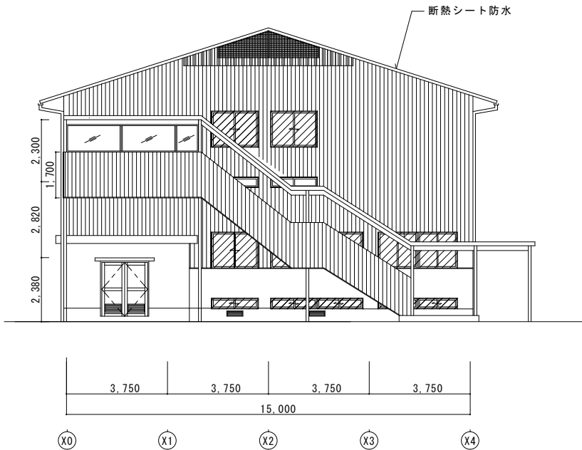
南側立面図 1/200
