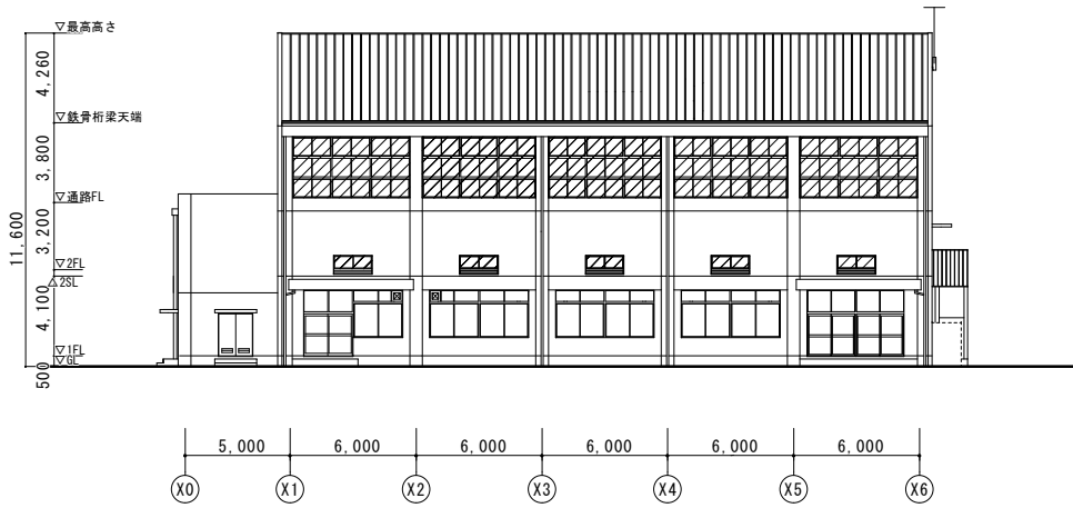
南側立面図 1/200
