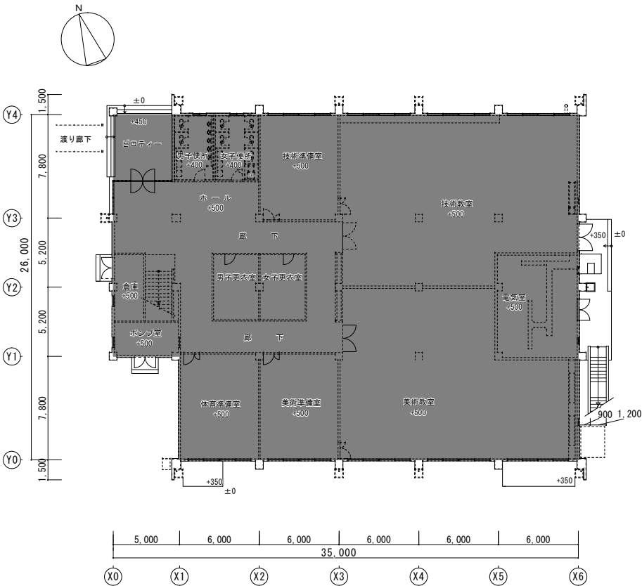
1階平面図 1/200
