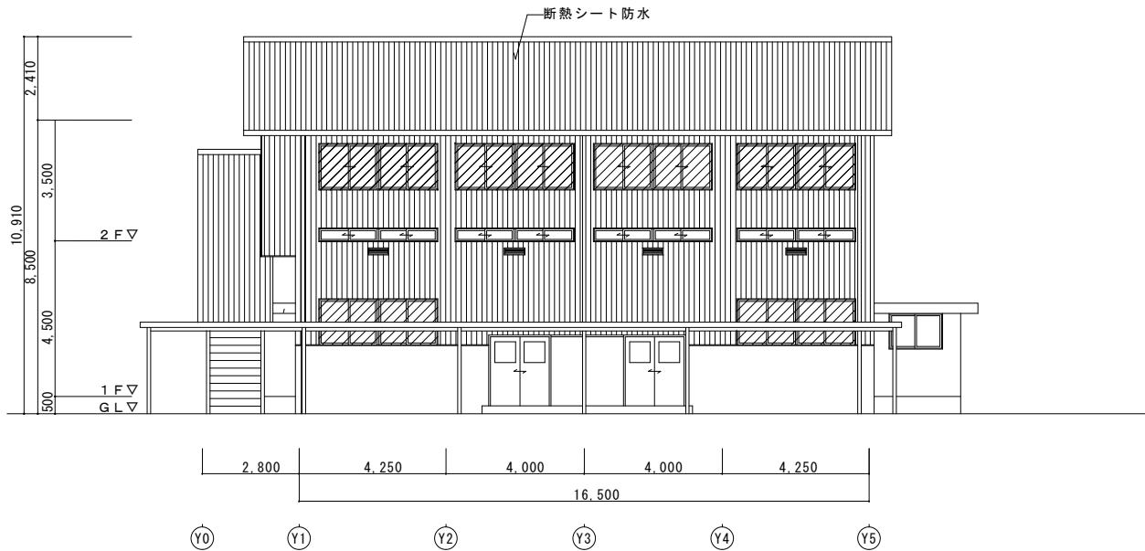
東側立面図 1/200
