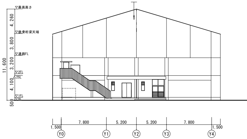
東側立面図 1/200
