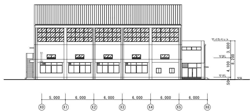
北側立面図 1/200
