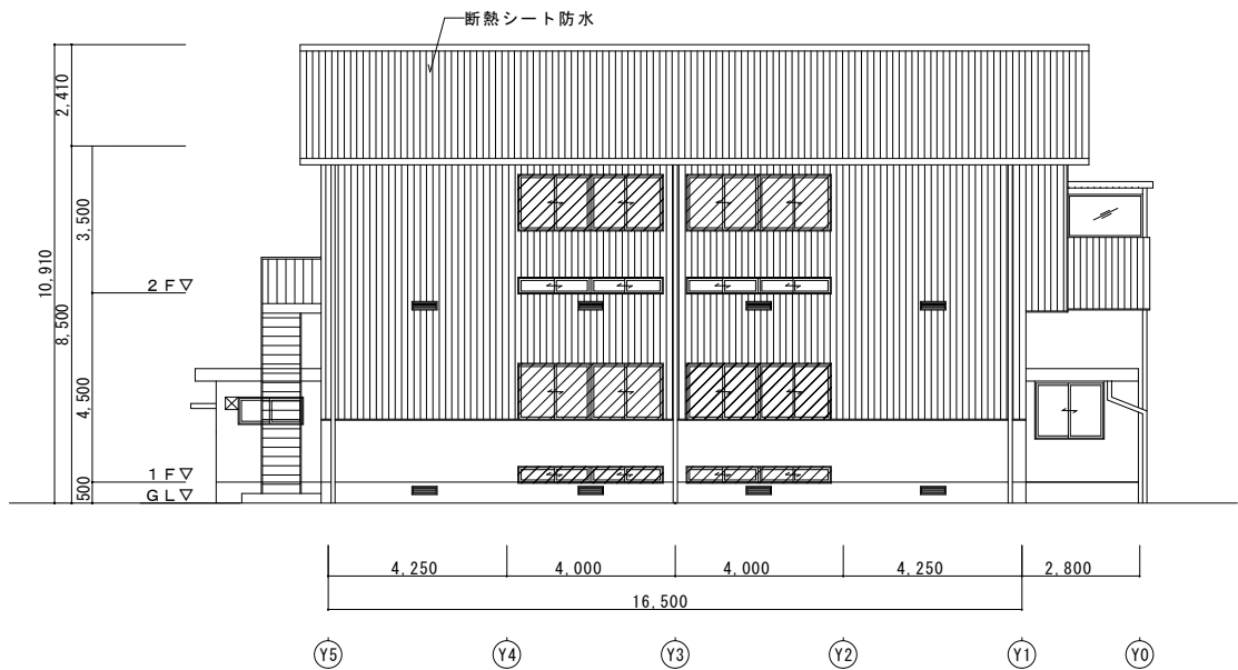
西側立面図 1/200
