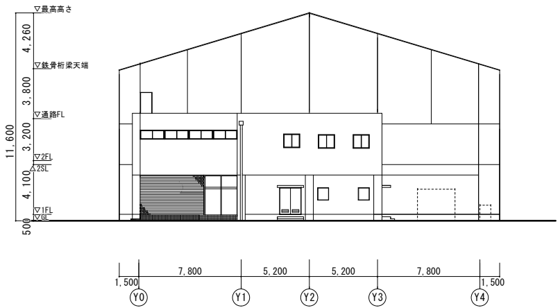
西側立面図 1/200
