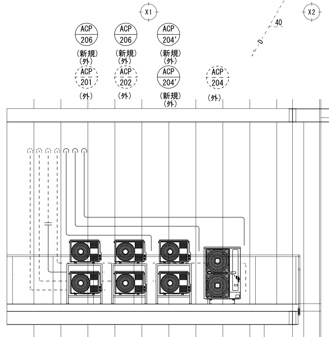
2階平面図 (改修後)
