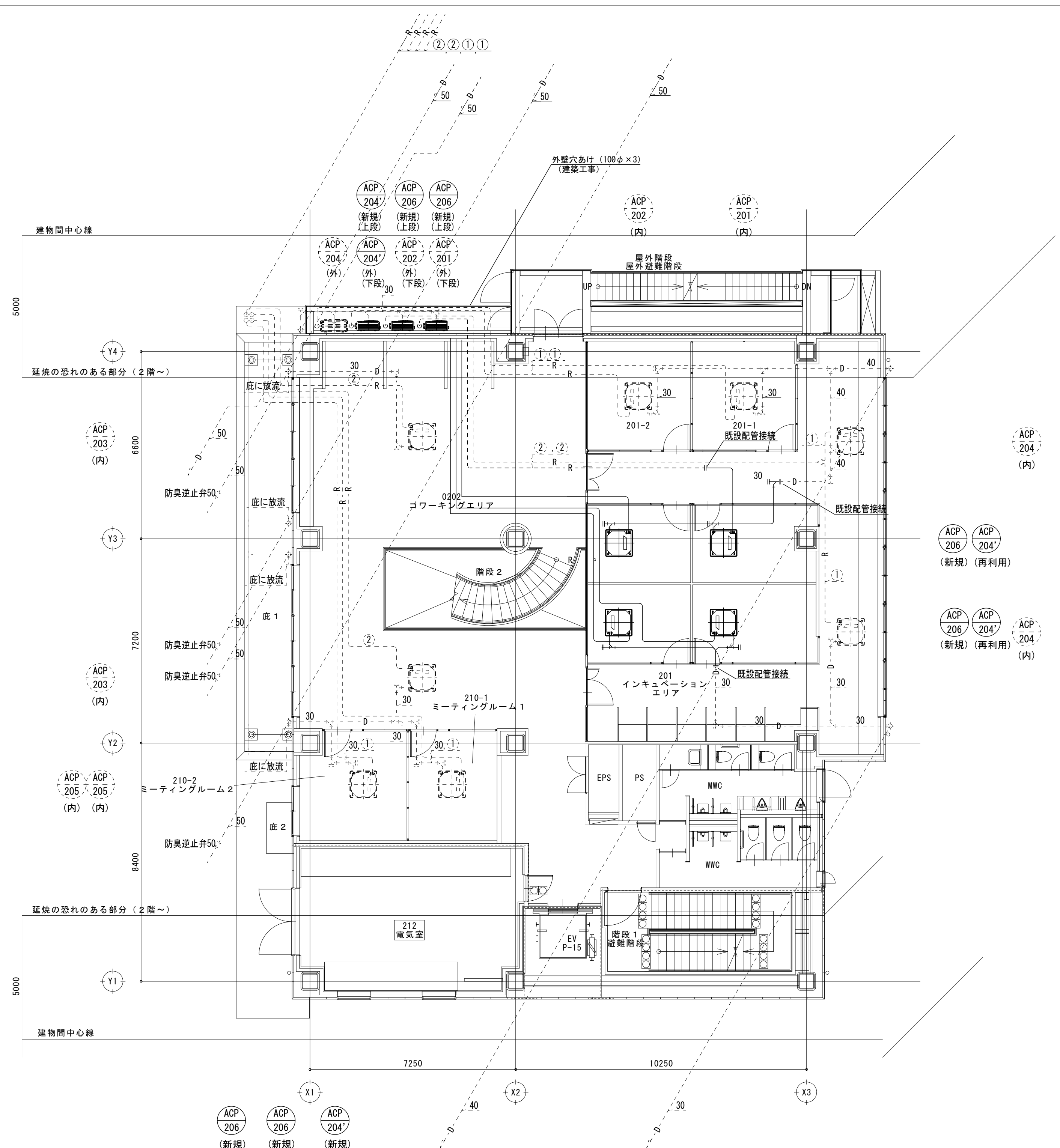
2階平面図 (改修後)
